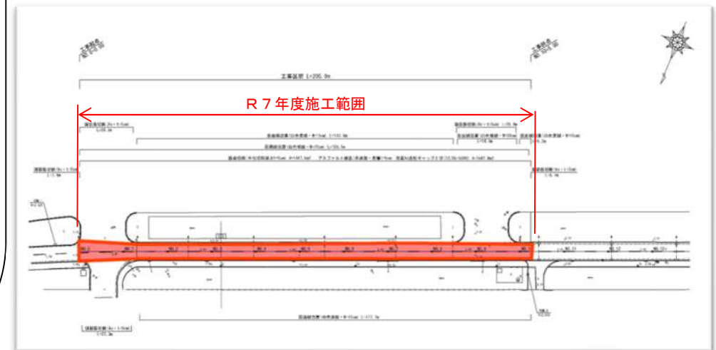
平面図
